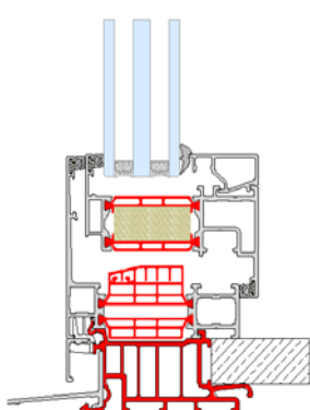
Basis profiel verdoken ontwatering Profil d'appui isolante drainage invisible
